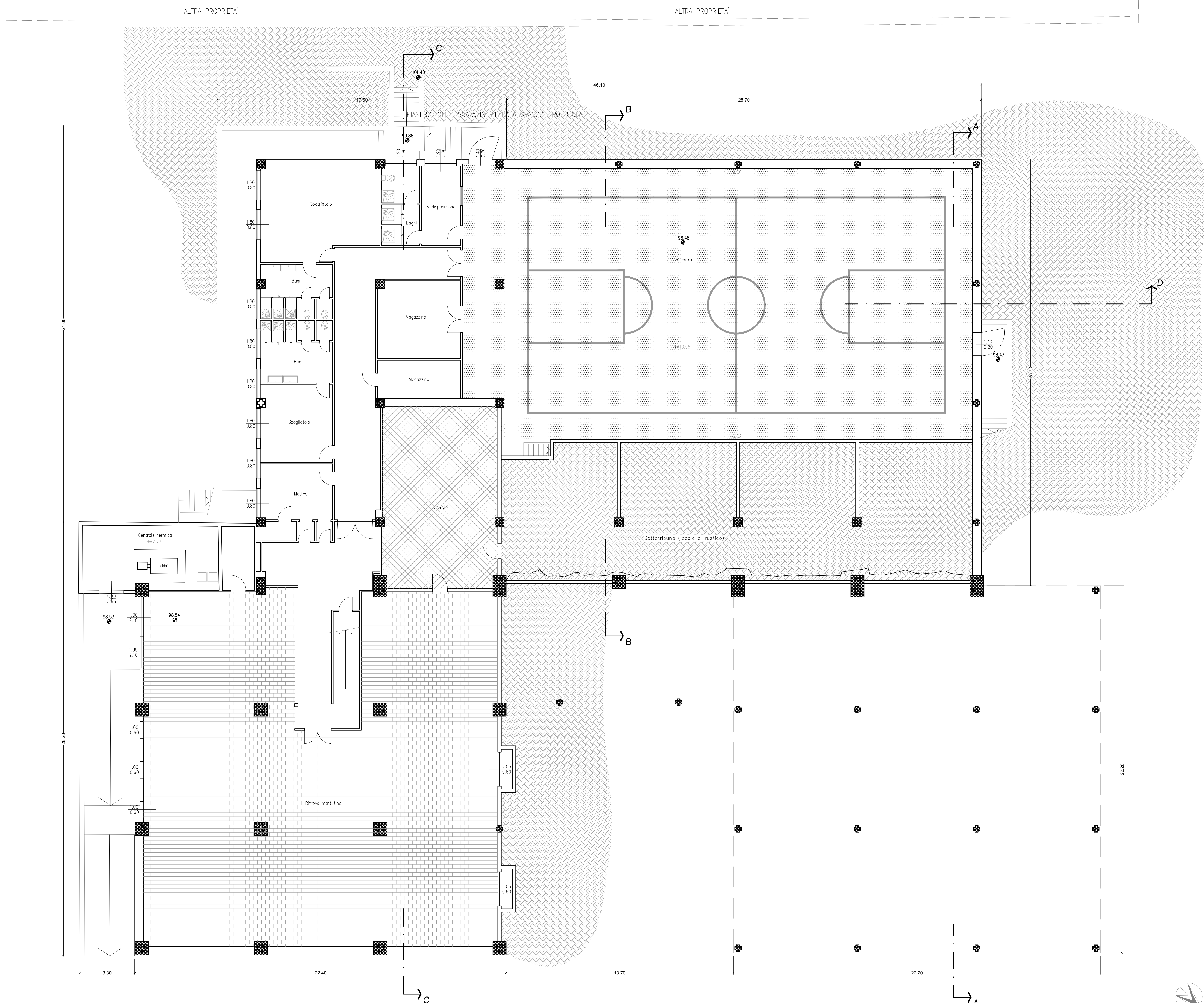
PIANTA PIANO INTERRATO scala 1:100
