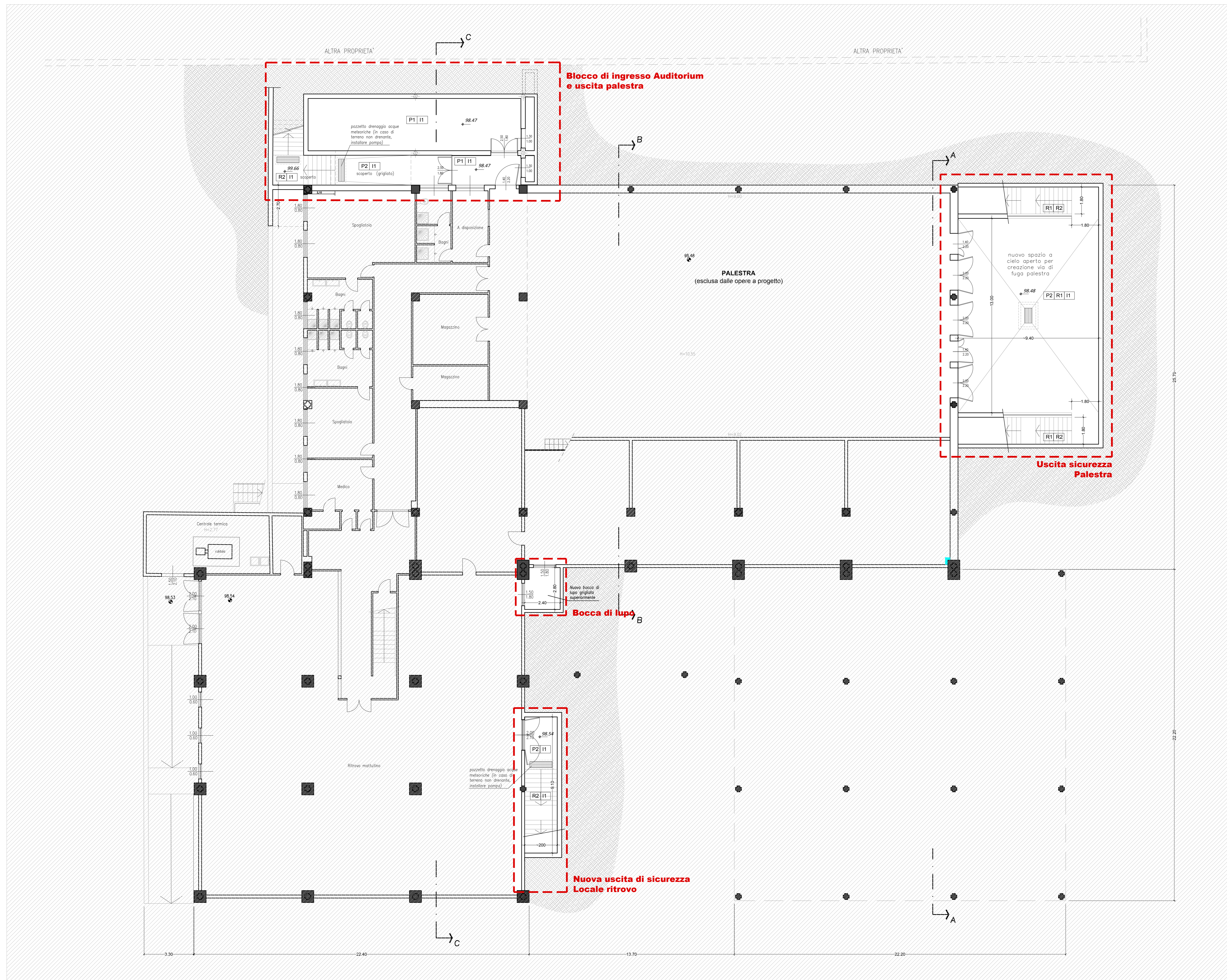
PIANTA PIANO INTERRATO scala 1:100
