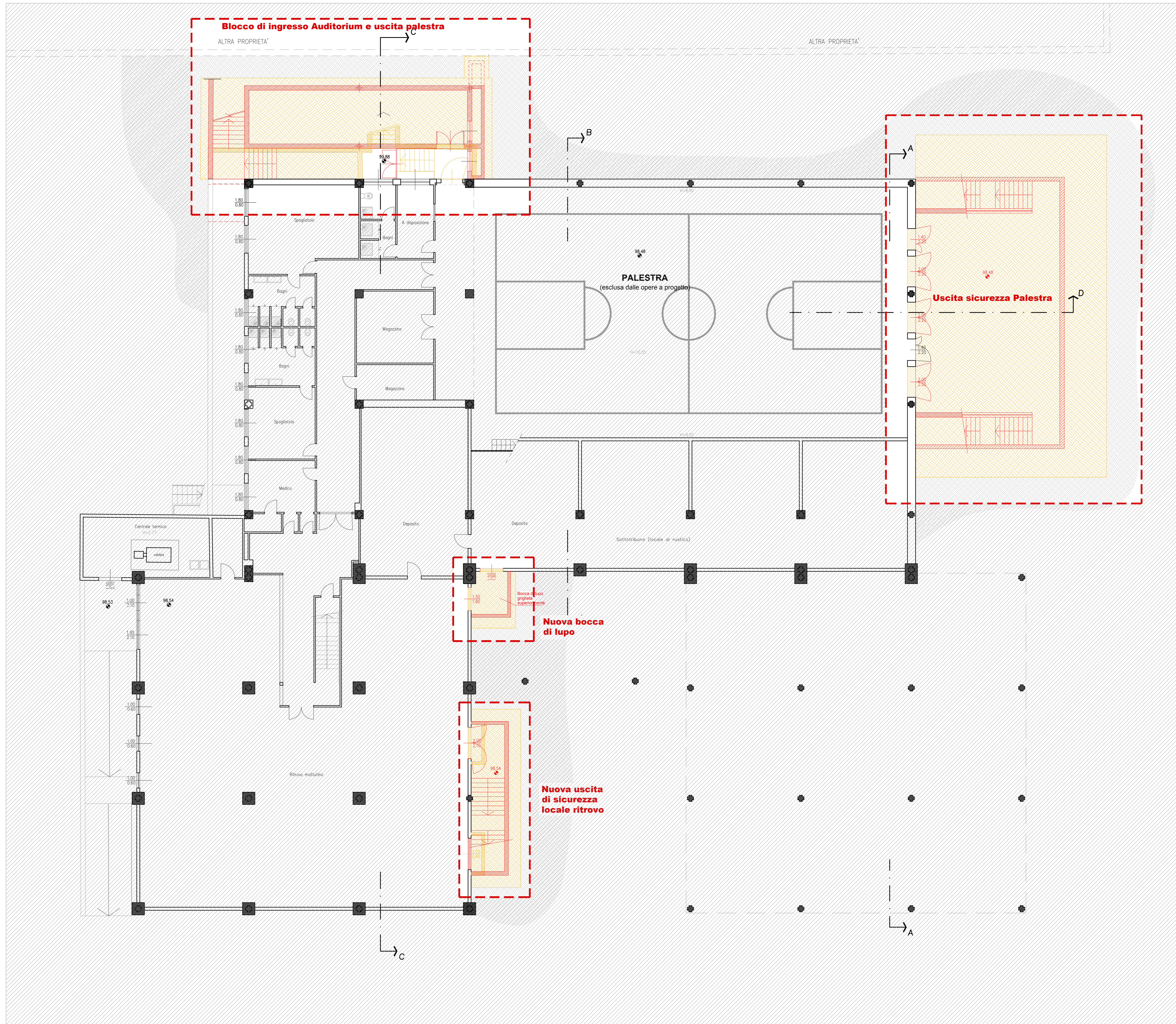
PIANTA PIANO INTERRATO scala 1:100
