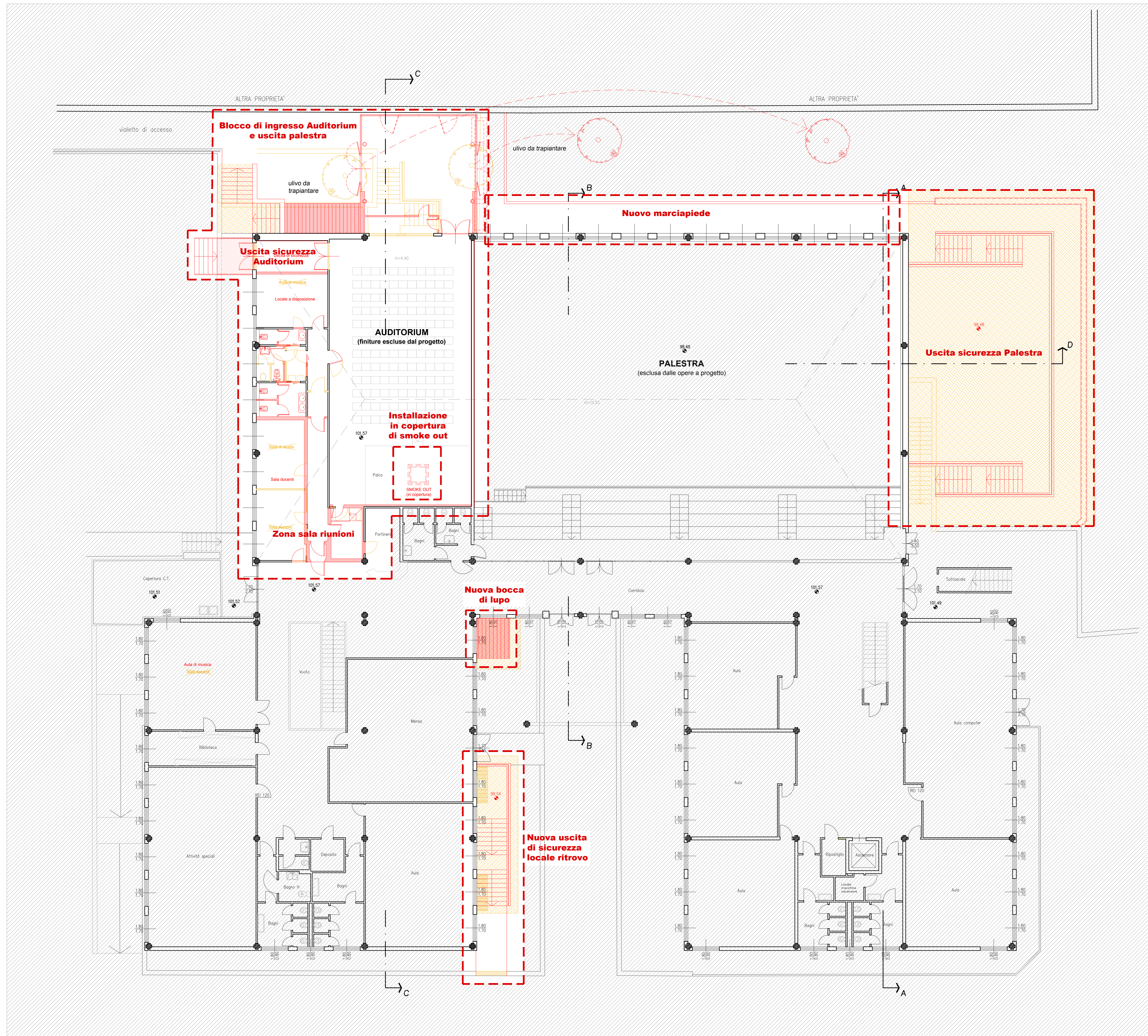
PIANTA PIANO TERRA scala 1:100
