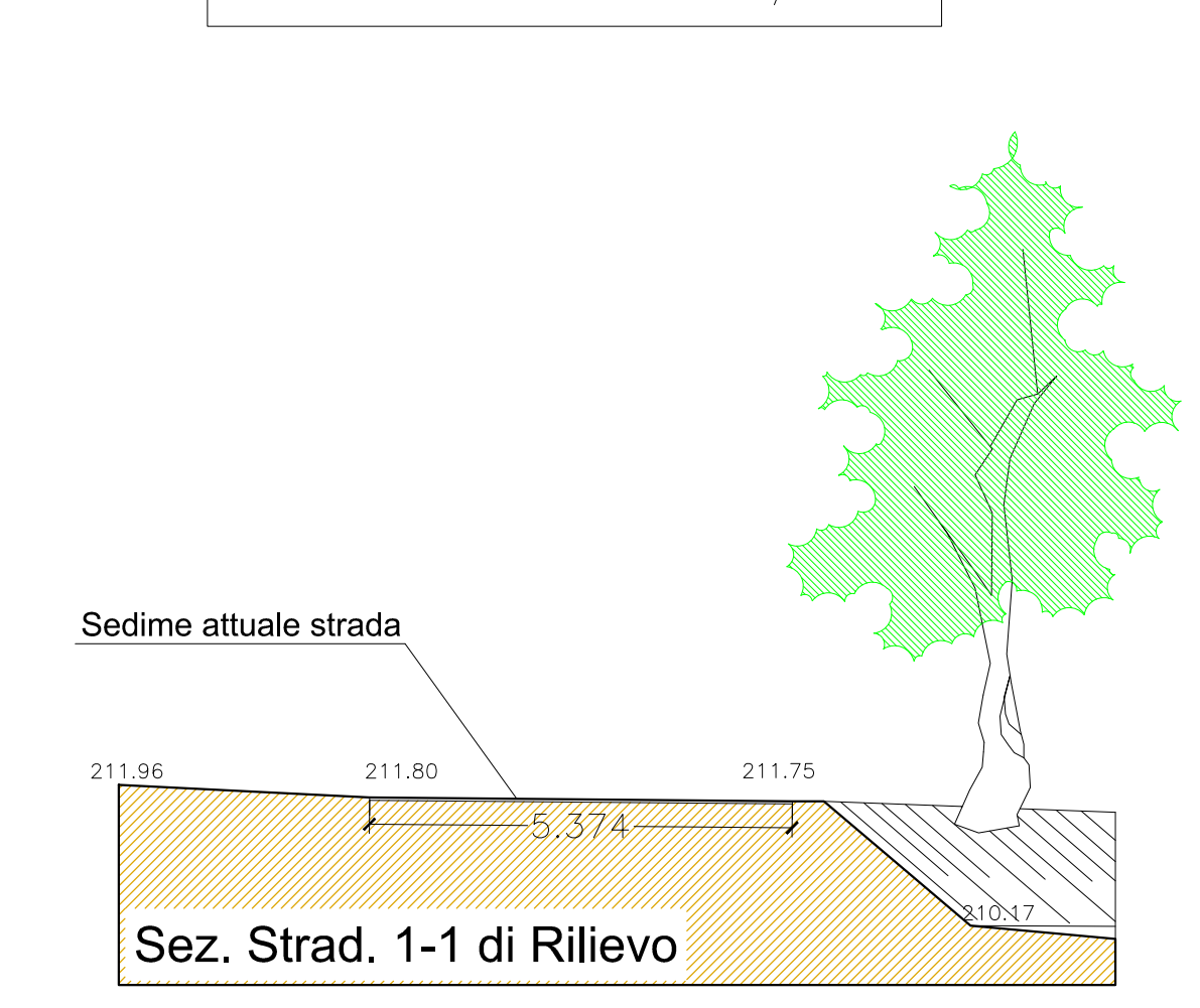
Sezione Della Strada Di Rilievo Scala 1/100
