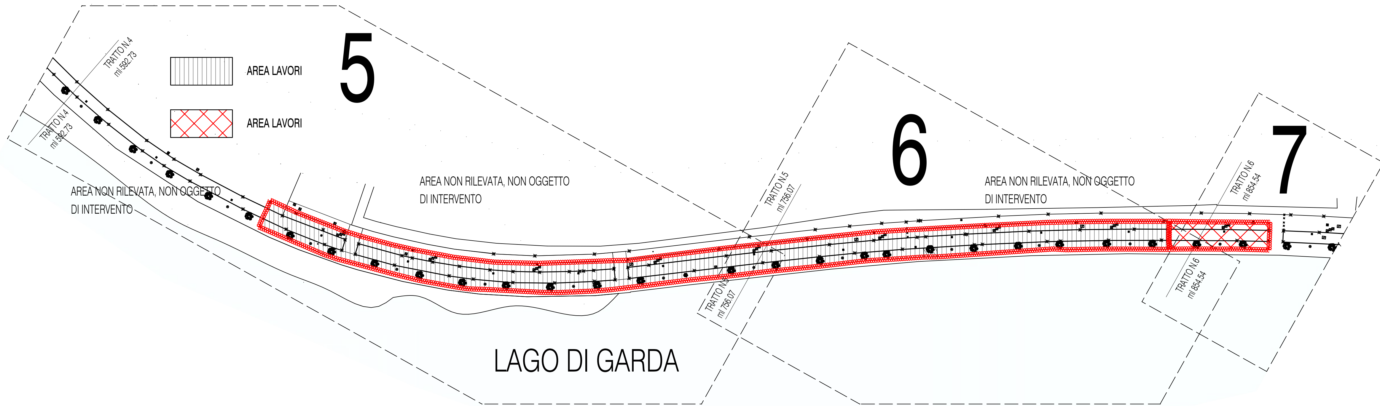
PLANIMETRIA GENERALE DI CANTIERE COMPLETA: AREA LAVORI + AREA CANTIERE SCALA 1:500
