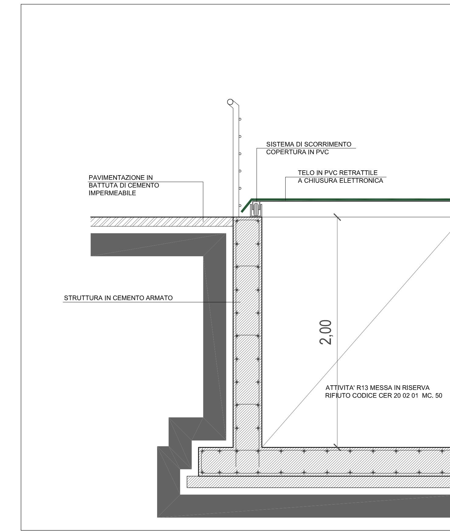
PARTICOLARE COSTRUTTIVO "A" - AREA MESSA IN RISERVA RIFIUTI Scala 1:20
